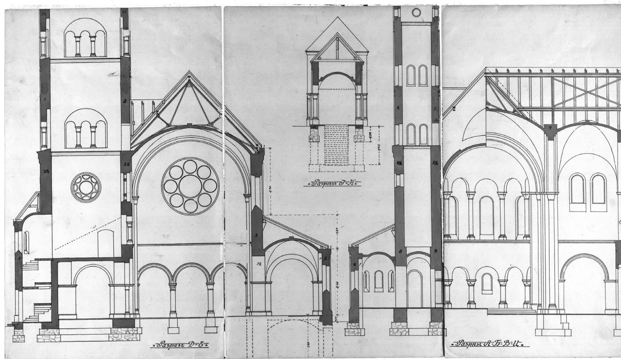
Ил. 24. Технический план постройки костела Святых Сымона и Елены в г. Минске (фрагмент), 1905 г.
